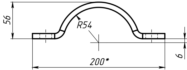
Поз.4 (Полухомут)
