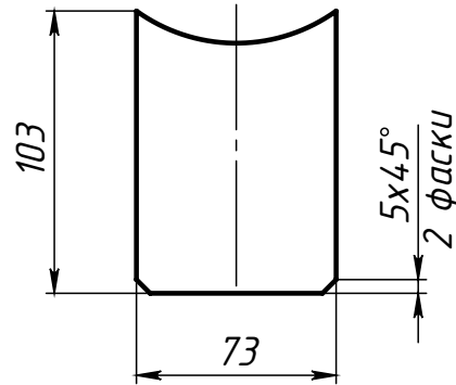
Поз.3 (Ребро)
